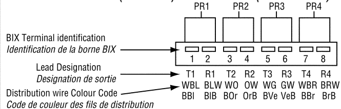
Modular Jack Front View — TIA/EIA T568A (ISDN) Connecteur modulaire - vue de face — TIA/EIA T568A (RNIS)
